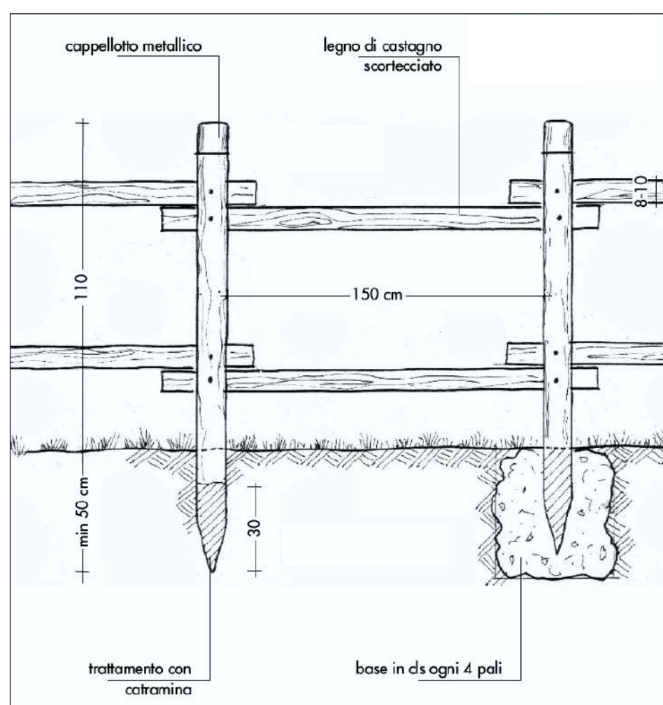
Staccionata tipo: legno di castagno
