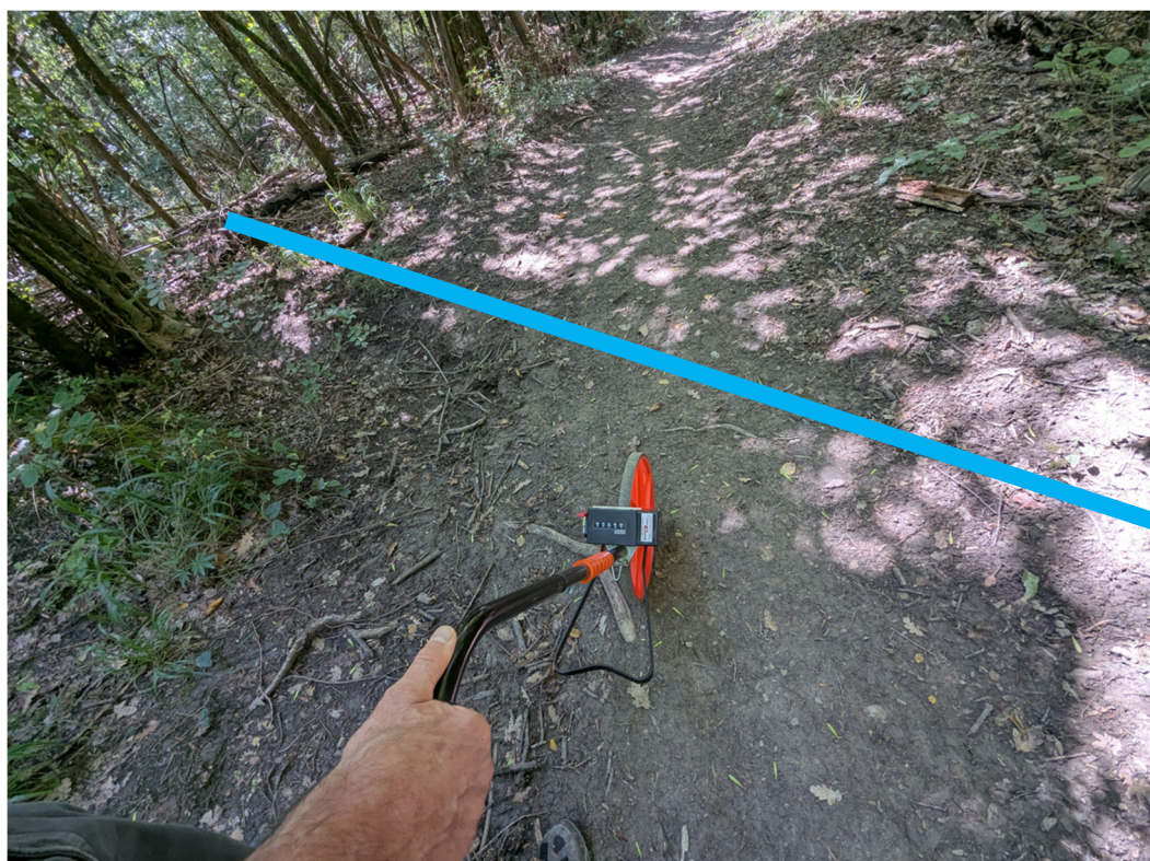
Foto 9 – Progressiva 222,0m = traversa taglia acqua in progetto
