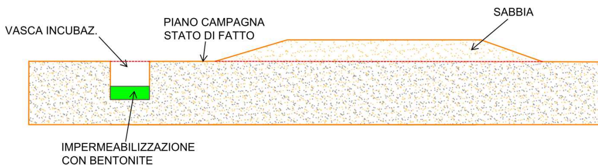
Figura 1 – Sezione tipo del sito di riproduzione
