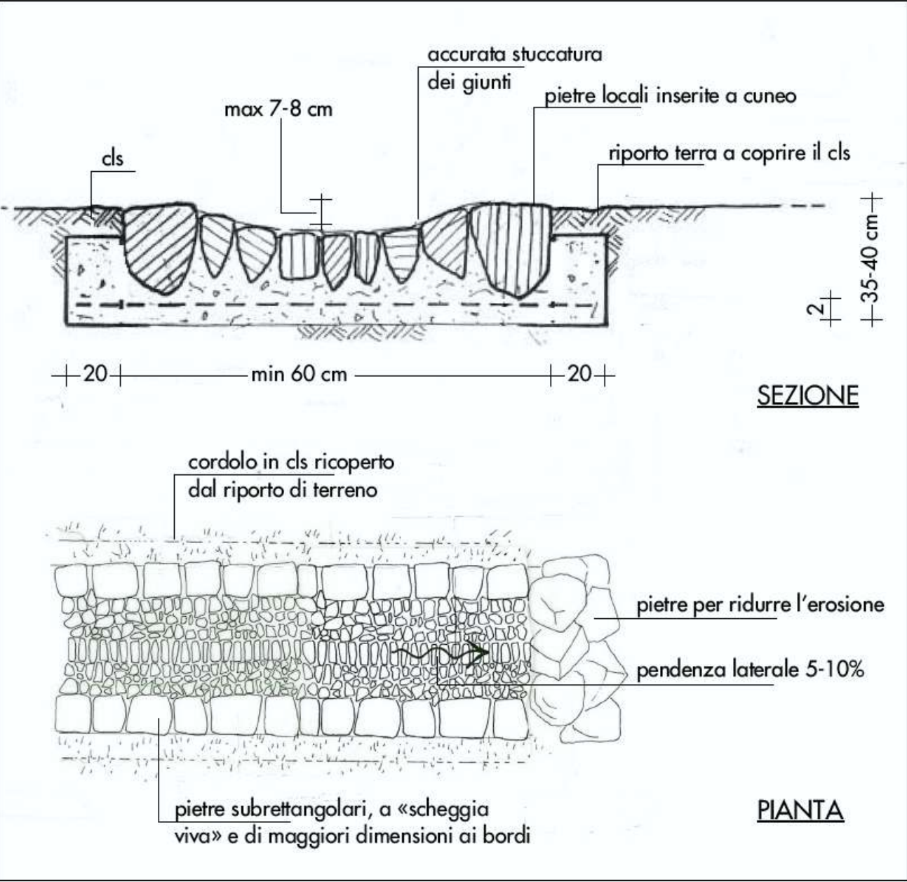
Basto in pietra per lo sgrondo delle acque
