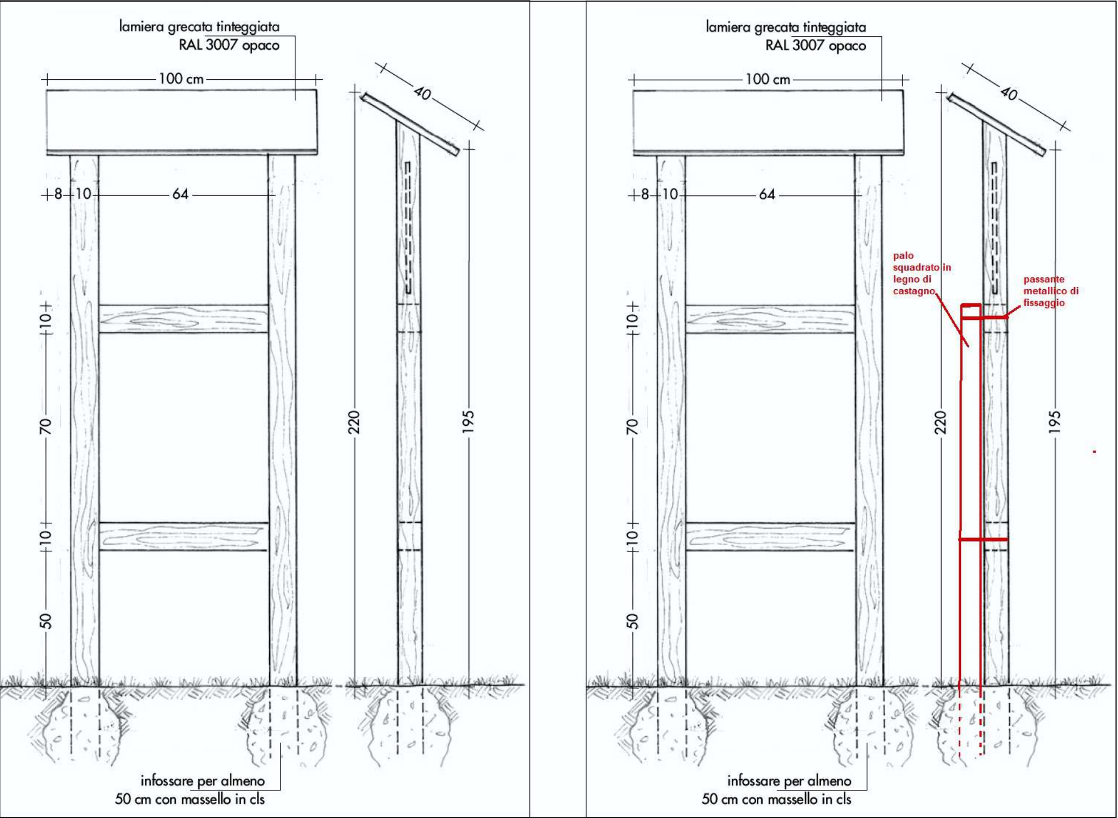
Tipologia nuova bacheca per cartelli didattici e consolidamento bacheca esistente
